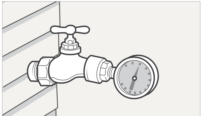
Abbildung 1: Zur Prüfung des Wasserdrucks montieren Sie ein Manometer an dem Außenhahn, der dem Wasserzähler am nächsten liegt. Ein Manometer erhalten Sie bei Ihrem Hunter-Händler vor Ort.
