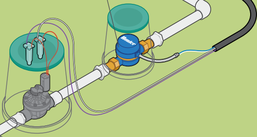
Durchflussüberwachung HC-Durchflussmessgerät
